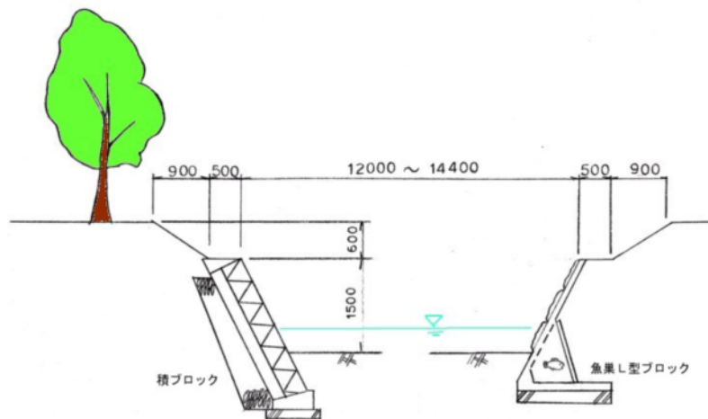
標準断面図
